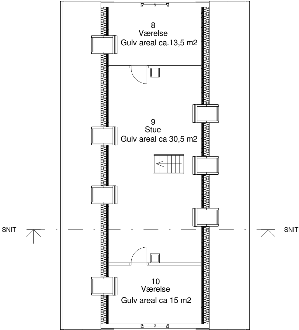
Samlet beboelsesareal af tagetage målt udv. kant tag 1,5 m over O.K. gulv ca. 67,5 m2
