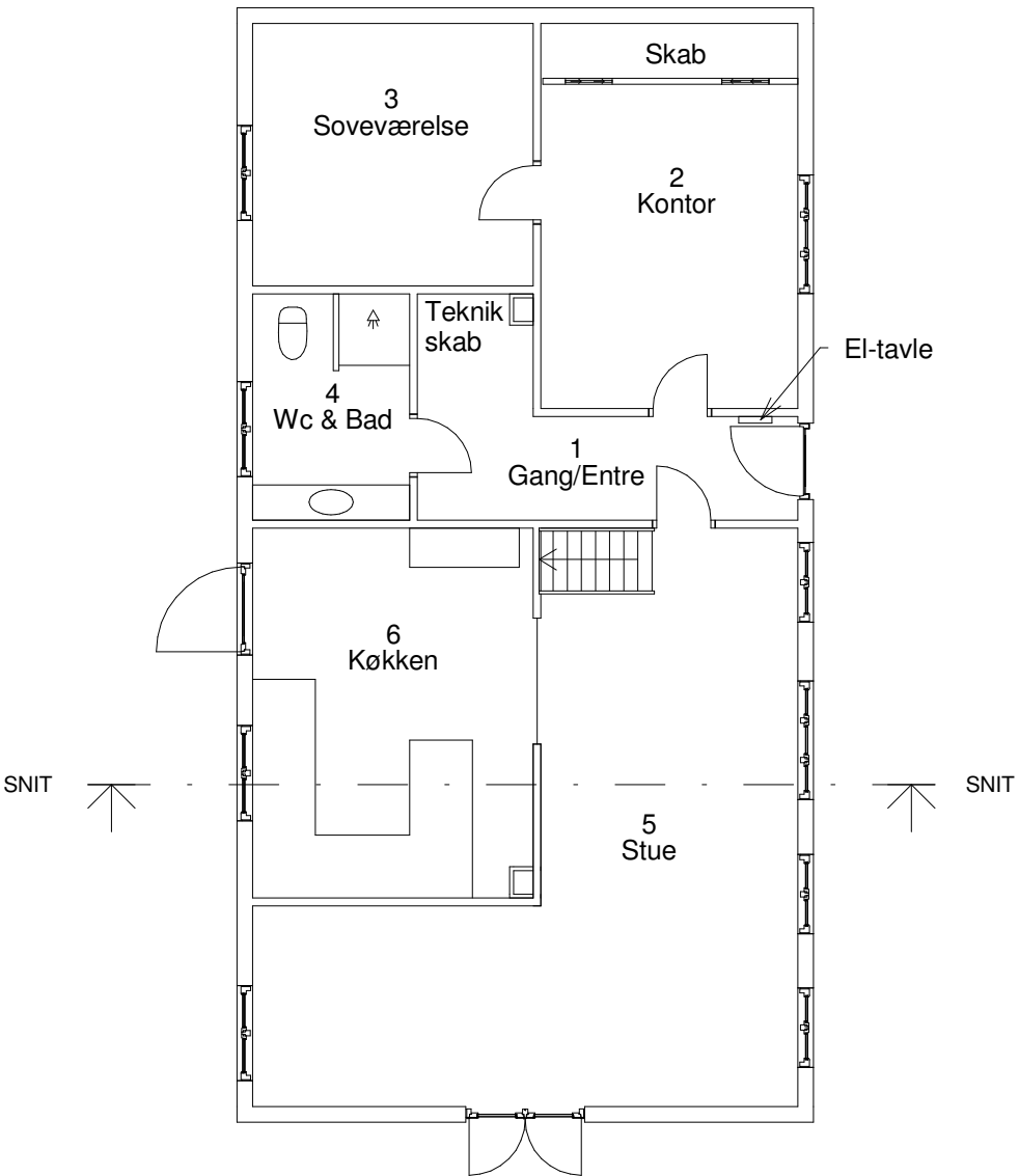
1 02_STUE 1 : 100
